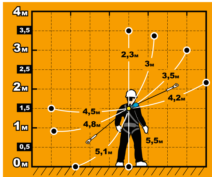
Рис. 10 Расчет минимальной высоты (запаса высоты) рабочего места в зависимости от положения анкерного устройства относительно пользователя.
