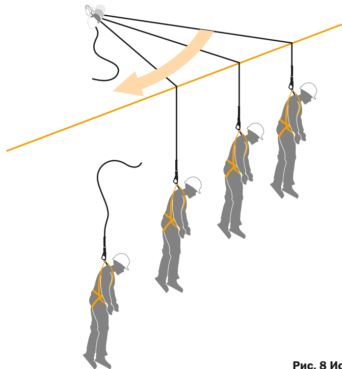
Рис. 8 Истирание троса до разрыва при падении с маятниковым перемещением.
