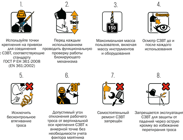
Рис. 2 Этикетка с маркировкой и обозначение пиктограмм.
